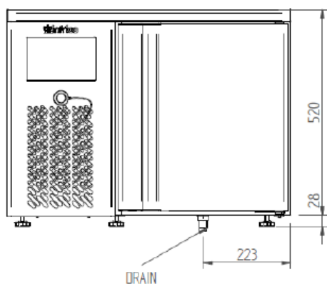
ALZADO
