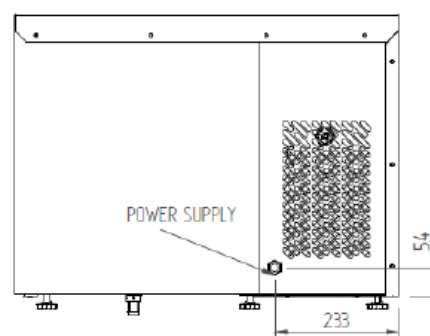
TRASERA
