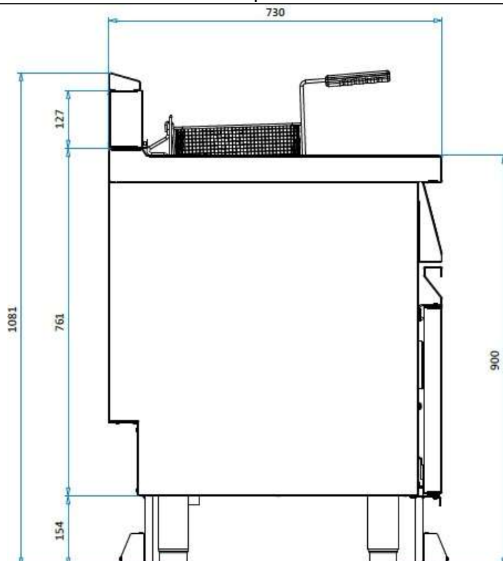
Dessin technique - vue latérale
